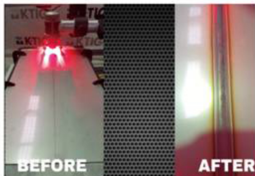
용접 전후 대비 2mm 서스 평판 용접
