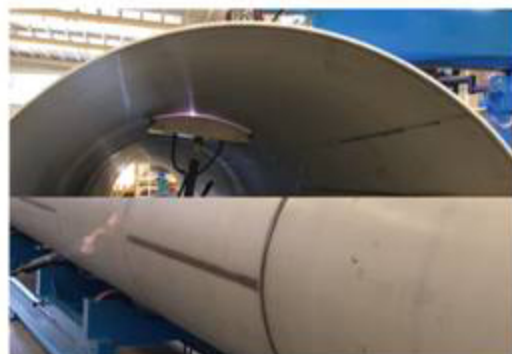
길이 12m, 직경 1.6m 304스스 9mm의 대형 파이프 공정
