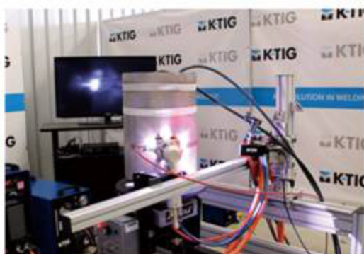
2G 용접 (2G welding) 304서스 4.2mm에 용접 실행
